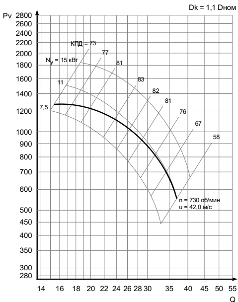
Рис. 12в - Dk=1,1 \text{ Дном}
