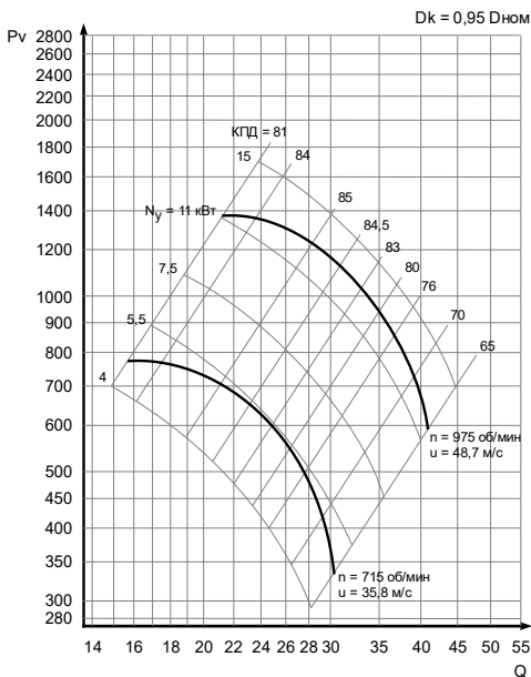
Рис. 12а - Dk=0,95 \text{ Дном}
