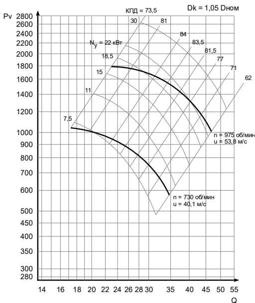
Рис. 12б - Dk=1,05 \text{ Дном}
